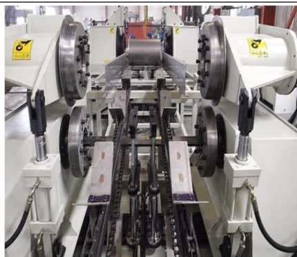
两辊卷板机
